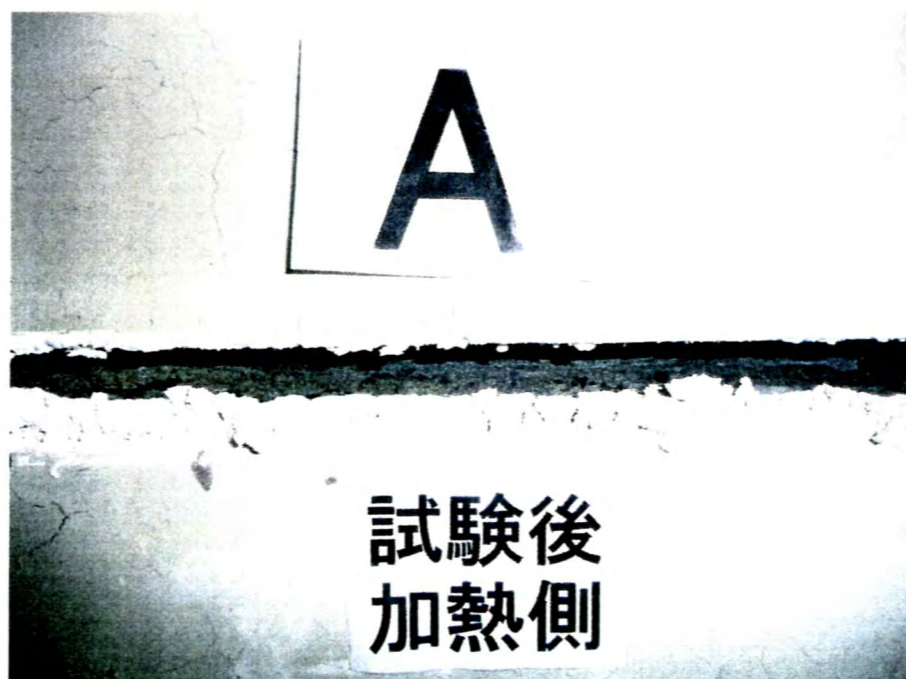
写真-14 試験後の水平スリット部（加熱側，屋外側）の状況 （試験体記号A）
