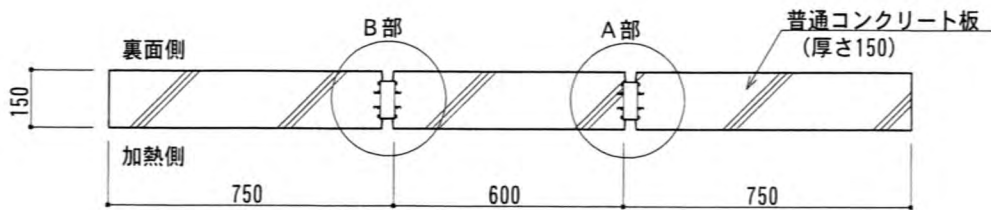
水平断面図
