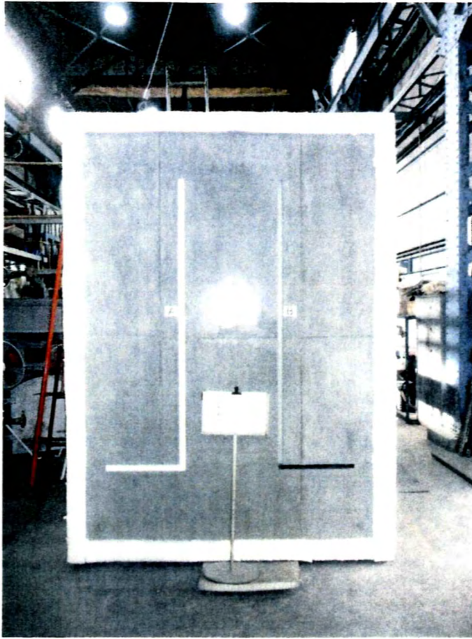
写真-1 試験前の加熱側の状況
