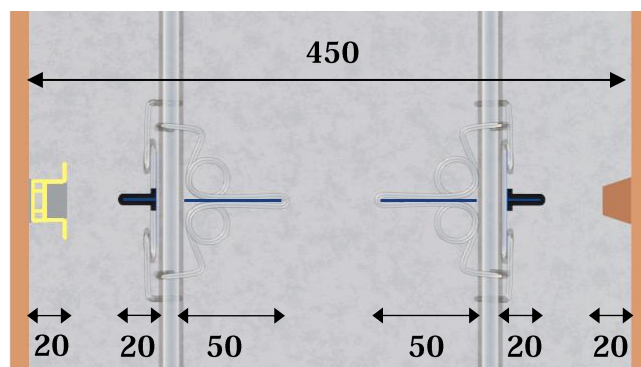
断面欠損率の算定方法(例)
