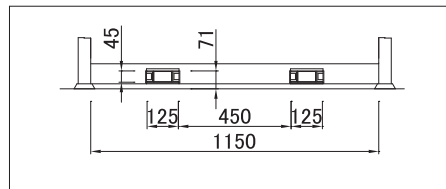
ツメ位置詳細図
