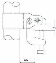
スイッチクランプ
