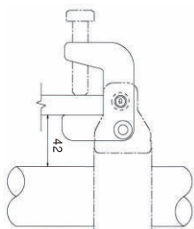
スイッチクランプ
