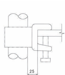
ガードクランプ
