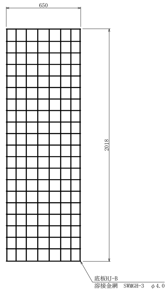
底板HJ-B平面図 S=1:10
