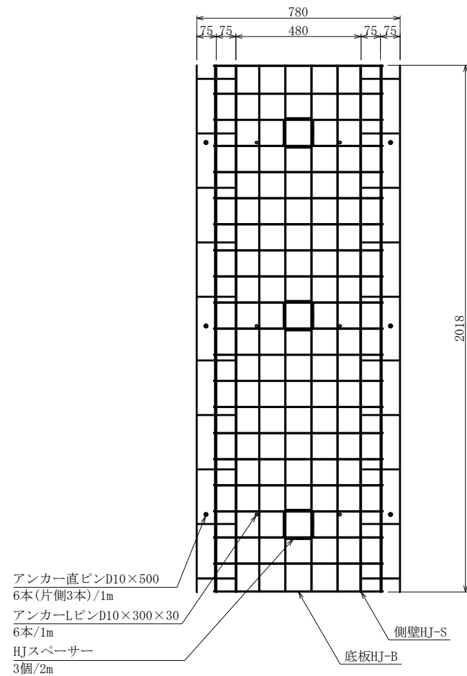
組合せ平面図 S=1:10
