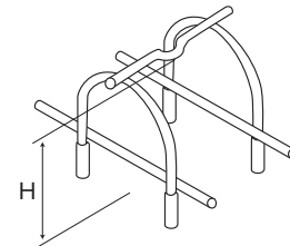
●S型 補強キャップ付
