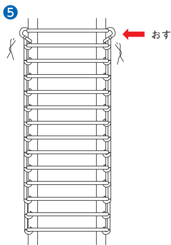
フープ筋の結束がおわったら持ちながらハンドル部の結束線を切りストッパーを外しながらハンドルを前に押してください。
