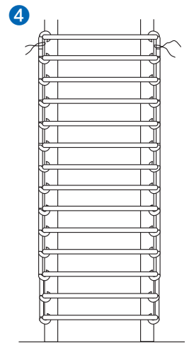
チェーンフックとフープ筋のセットがおわってから主筋とフープを結束してください。
