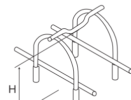
●W型 補強キャップ付
