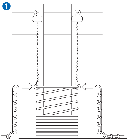
チェーンブロックを巻上げながら、チェーンフックに順次フープ筋をかけてゆく。
