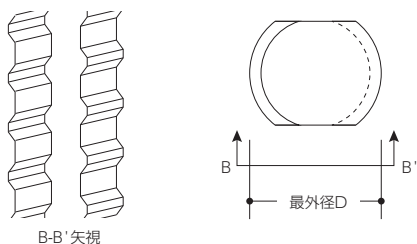
(b) 異形鉄筋(ねじ節)の一般的な形状
