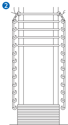
②・③・④・⑤と順にフープをセットしてください。
